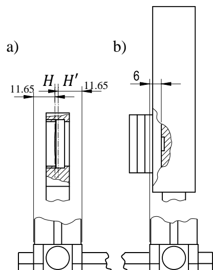
13 pav. a) Lęšio priekinės pagrindinės plokštumos H padėtis ir galinės pagrindinės plokštumos H' padėtis lęšio laikiklio kraštų atžvilgiu. b) Kameros CCD matricos padėtis kameros laikiklio krašto atžvilgiu.
