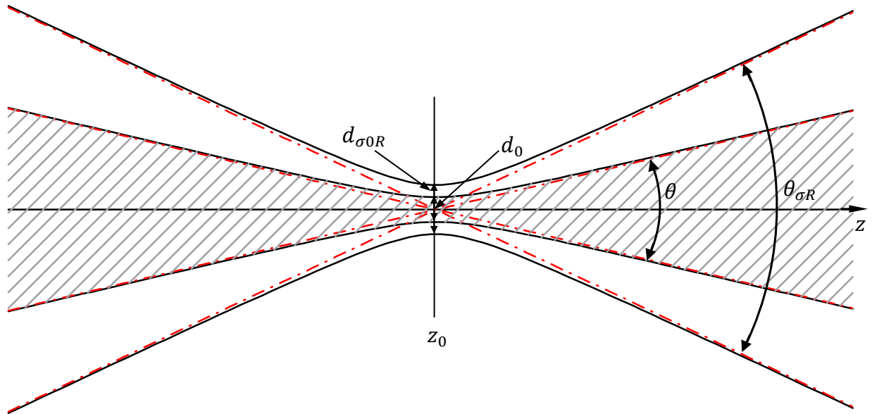
3 pav. Realus lazerio pluošto sklaidimas
